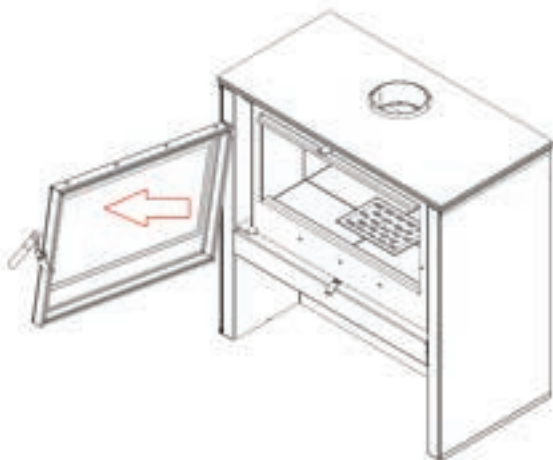
16. Schemat wymiany drzwi JUNGLE / The JUNGLE door-replacement diagram
