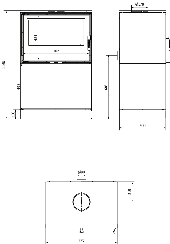
81. Zwymiarowany rysunek pieca KARI Dimensioned Figure of the KARI Maßzeichnung des Ofens KARI Рисунок камина KARI с определением размеров.
