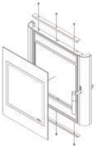
35. Schemat wymiany szyby w piecu VEGA. The VEGA glass-replacement diagram
