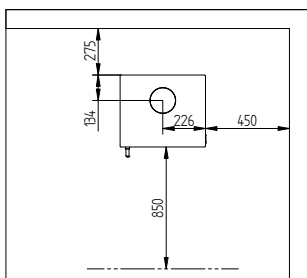
Avstånd till brännbart material utan isolerat röktör
