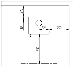
Abstand zu brennbarem Material ohne isoliertes Rauchrohr
