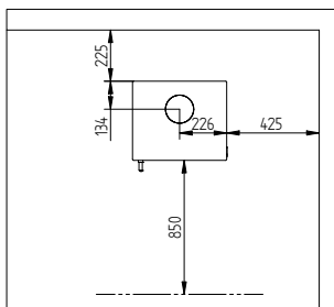
Afstand til brændbart materiale med isoleret røgrør
