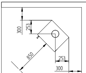
Abstand zu brennbarem Material ohne isoliertes Rauchrohr
