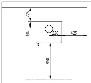
Avstånd till brännbart material med isolerat röktör
