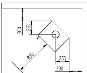
Afstand til brændbart materiale uden isoleret røgrør
