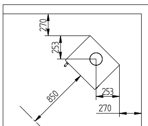
Afstand til brændbart materiale med isoleret røgrør
