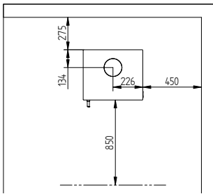
Afstand tot brandbaar materiaal zonder geïsoleerde kachelpijp
