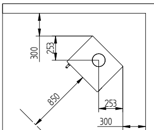
Afstand tot brandbaar materiaal zonder geïsoleerde kachelpijp
