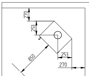
Avstånd till brännbart material med isolerat röktör
