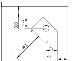
Avstånd till brännbart material utan isolerat röktör
