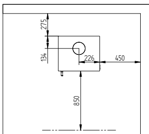
Afstand til brændbart materiale uden isoleret røgrør
